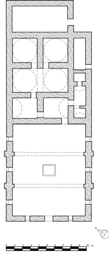
Çizim 4: Hamam-ı Cedid, plan. (Çuhadaroğlu ve Oğuz 1975:72)
