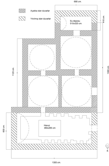
Çizim 17: Hasan Ağa Tekkesi Hamamı, kroki.
