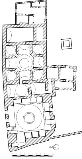
Çizim 2: Ömerge Hamamı, plan (Nicosia Master Plan 1979: 50).
