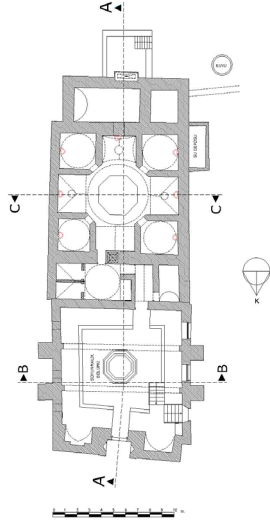
Çizim 1: Büyük Hamam, plan (Vakıflar Genel Müdürlüğü İnşaat Şubesi'nden alınmıştır).
