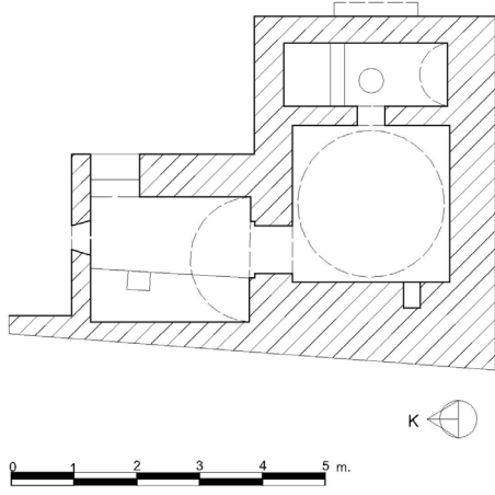
Çizim 16: Şömineli Ev Hamamı, plan.
