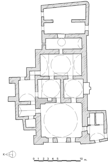
Çizim 4: Mehmet Bey Ebubekir Hamamı, plan (Bilgilendirme levhasından alınarak ölçeklendirilmiş ve yeniden işlenmiştir).
