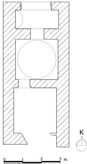
Çizim 14: Hisarköy Hamamı, plan.
