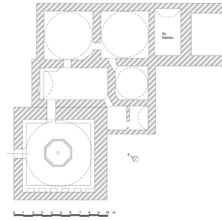
Çizim 13: Kızıl Hamam, restitüsyon.
