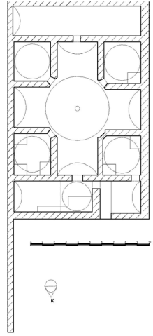
Çizim 9: Tandi'nin Hamamı, plan.
