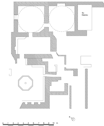
Çizim 12: Kızıl Hamam, plan.
