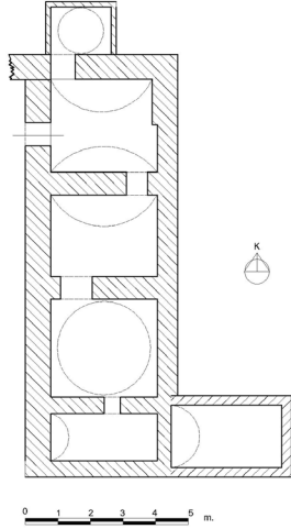
Çizim 8: Muslu Çavuş Hamamı, plan.
