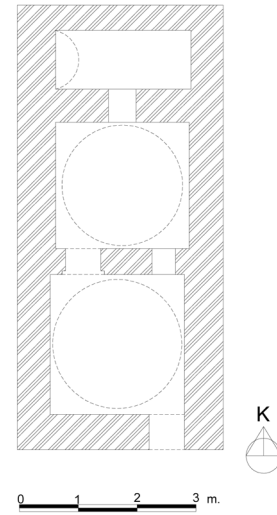
Çizim 15: Hisarköy Hamamı, restitüsyon.
