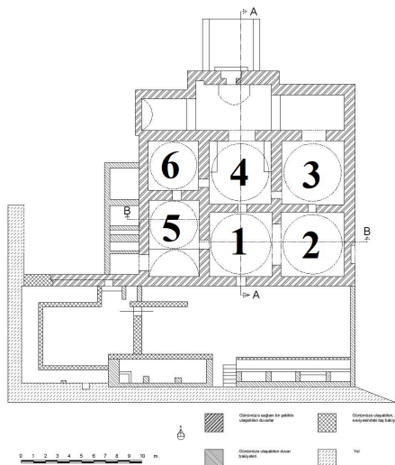
Çizim 10: Keltikli Hamam, plan.
