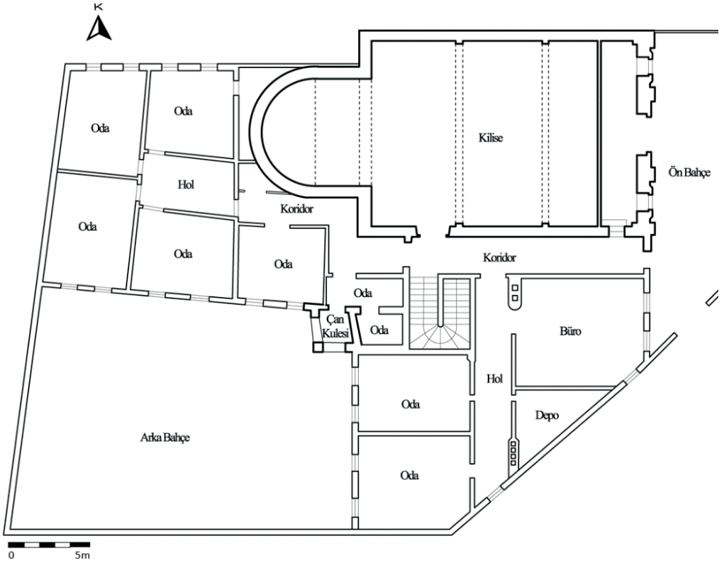
Plan 2: Samsun Mater Dolorosa Katolik Kilisesinin Planı 56
