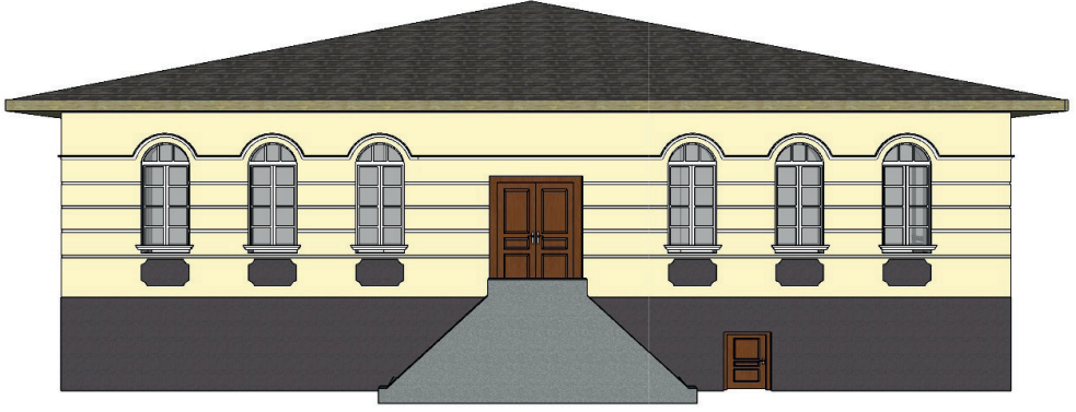
Çizim 2: Hisarköy İlk Mektebi Kuzeybatı Cephe Ayağa Kaldırma (D. Yönden & M. Ekmekci)
