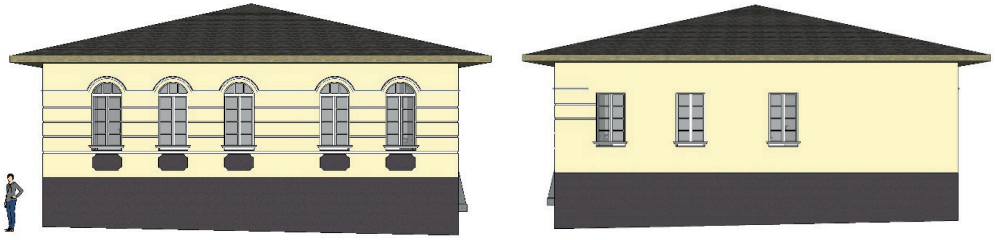
Çizim 3: Hisarköyü İlk Mektebi Kuzeydoğu ve Güneybatı Cephe Ayağa Kaldırma (D. Yönden & M. Ekmekci)
