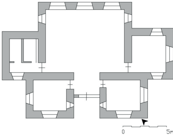
Çizim 2: Gürün Rüştîyesi muhtemel orijinal planı (Hacer Zor Akın, SKVKBK'den işlenerek)
