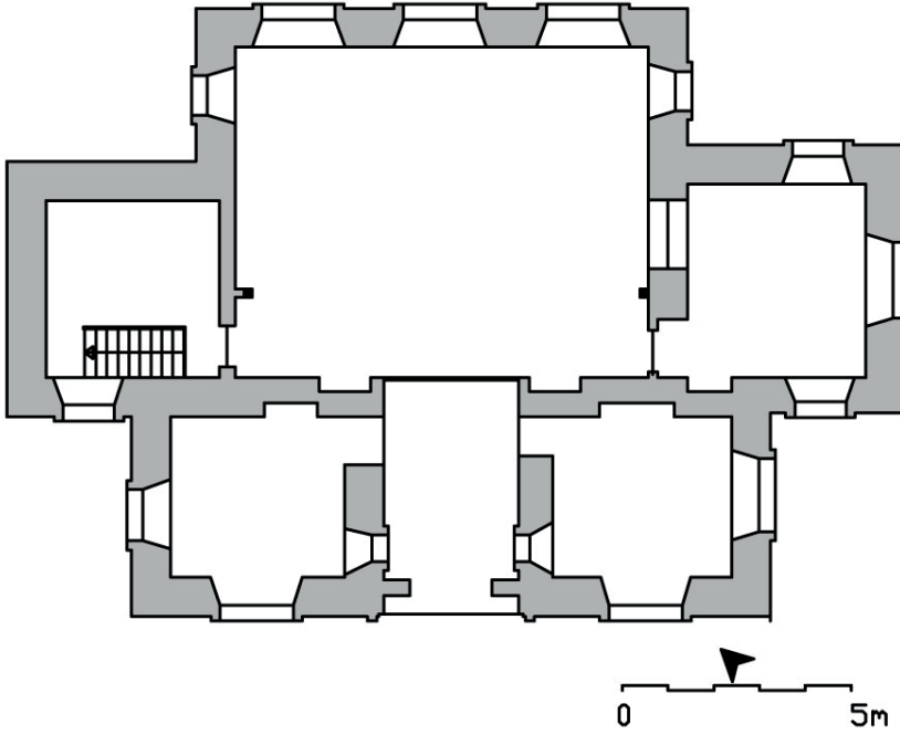
Çizim 1: Halk Kütüphanesi zemin kat planı (Hacer Zor Akın, Mimar Servet Çiftçi'den işlenerek)
