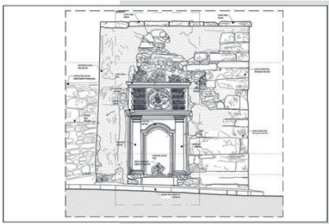
Şekil 3. Karagümruk Pertevniyal valide Sultan Çeşmesi çizim (Erişim tarihi: 04/02/2024. https://www.fatih.bel.tr/webfiles/userfiles/files/2_%20B%C3%96L%C3%9CM.pdf )
