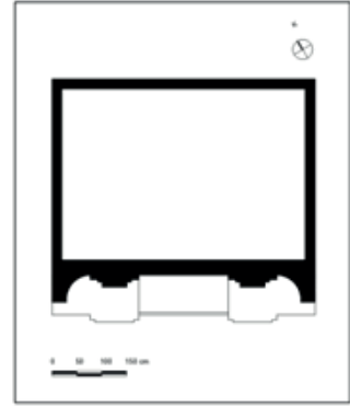
Şekil 2. Çeşmenin planı
