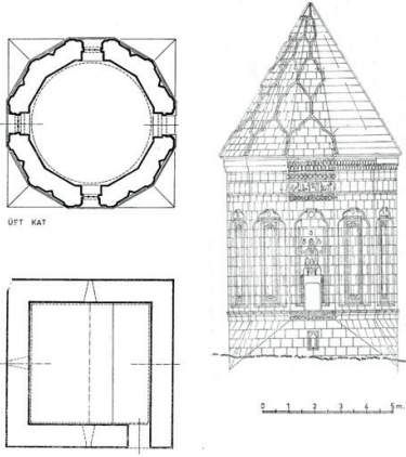
Çizim 25: Gevaş Halime Hatun Kümbeti (Tuncer, 1992)
