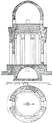
Çizim 14: Hasankeyf Zeynel Bey Türbesi (Yurttaş, 1996)
