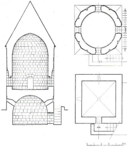
Çizim 24: Ahlat Erzen hatun Kümbeti (Tuncer, 1991)
