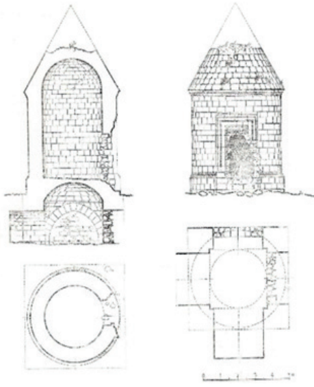
Çizim 10: Kemah Togay Hatun Kümbeti (Tuncer, 1991)
