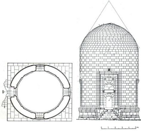
Çizim 12: Kayseri Sırçalı Kümbet (Tuncer, 1992)
