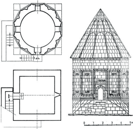
Çizim 28: Erciş Kadem Paşa Kümbeti (Tuncer, 1992)
