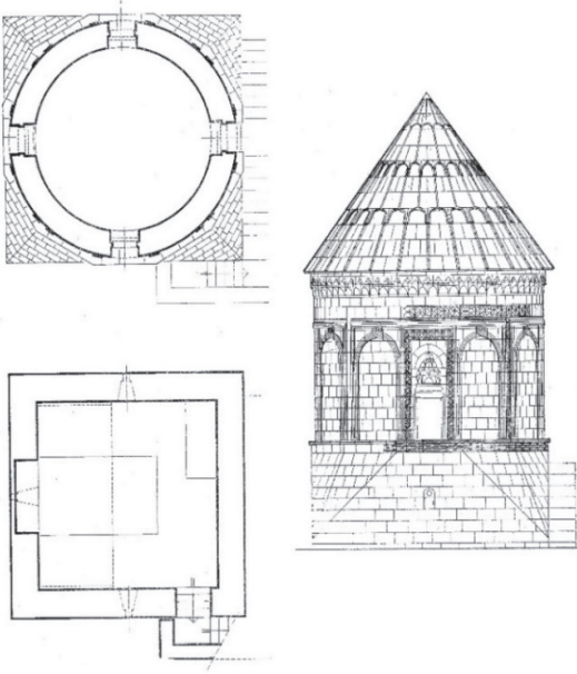
Çizim 5: Ahlat Bugatay Aka Kümbeti (Tuncer, 1991)
