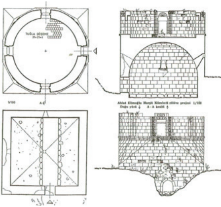
Çizim 4: Ahlat Alimoğlu Kümbeti (Tuncer, 1991)
