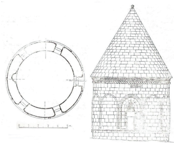
Çizim 7: Erzurum Silindirik Kümbeti (Tuncer, 1991)
