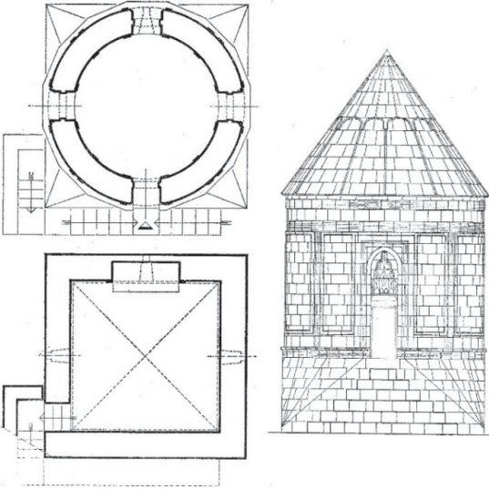
Çizim 2: Ahlat Hüseyin Timur Kümbeti (Tuncer, 1991)
