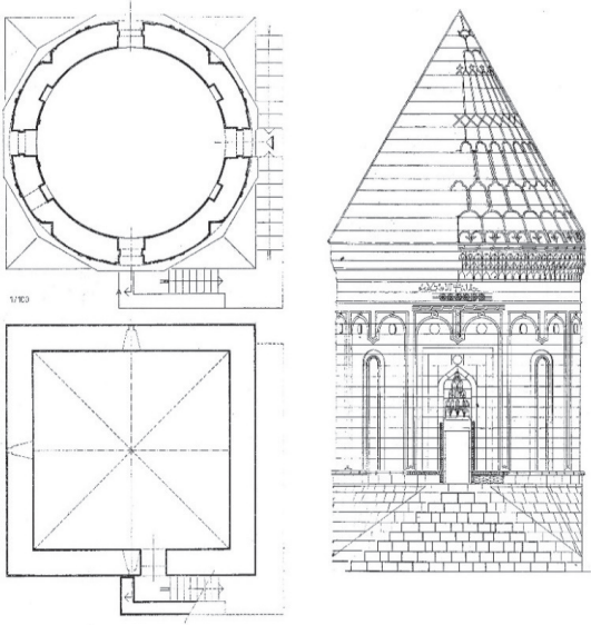
Çizim 3: Ahlat Usta Şagirt Kümbeti (Tuncer, 1991)
