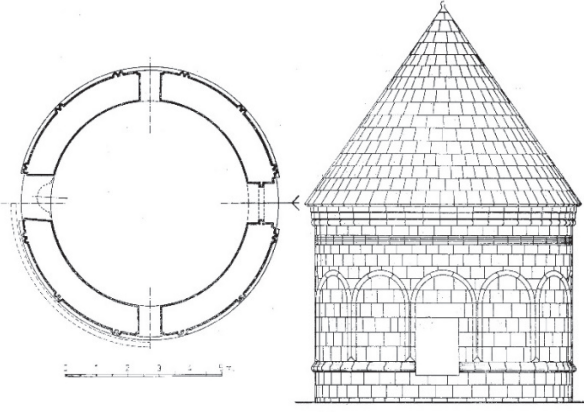
Çizim 8: Erzurum Cimcime Sultan Kumbeti (Tuncer, 1991)
