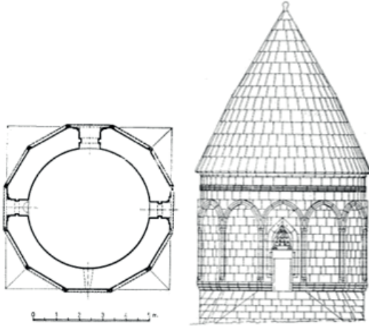
Çizim 20: Erzurum Onikigen Kümbet (Tuncer, 1991)
