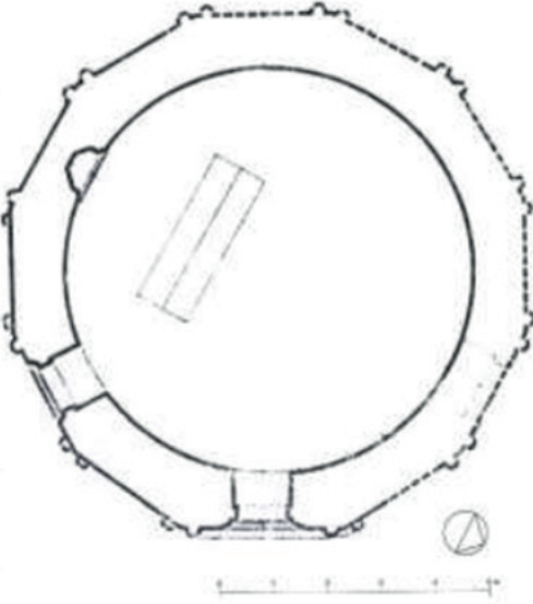
Çizim 21: Erzurum Rabia Hatun Kümbeti (Tuncer, 1991)
