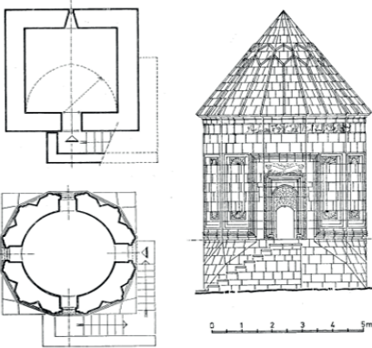
Çizim 26: Erçiş Anonim Kümbeti (Tuncer, 1992)
