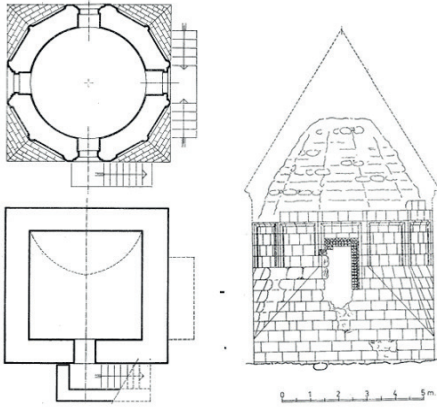
Çizim 27: Erciş Akçayuva Köyü Kümbeti (Tuncer, 1992)
