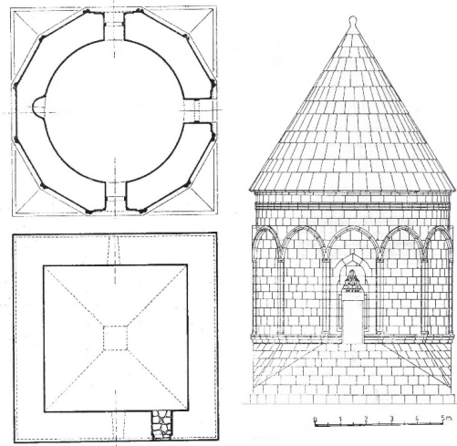
Çizim 19. Erzurum Gümüşlü Kumbet (Tuncer, 1991)
