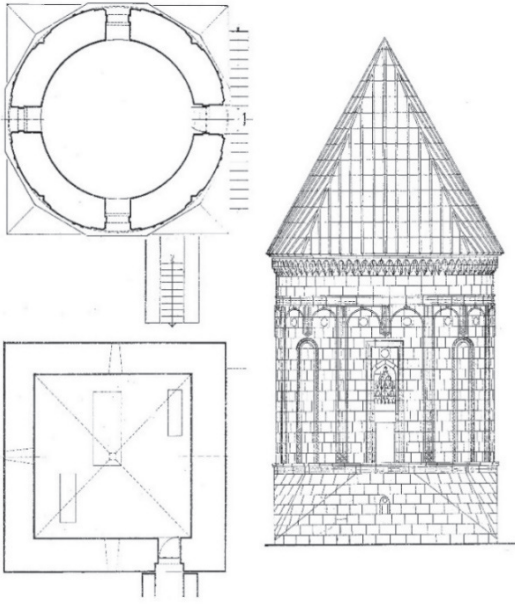
Çizim 1: Ahlat Hasan Padişah Kümbeti (Tuncer, 1991)
