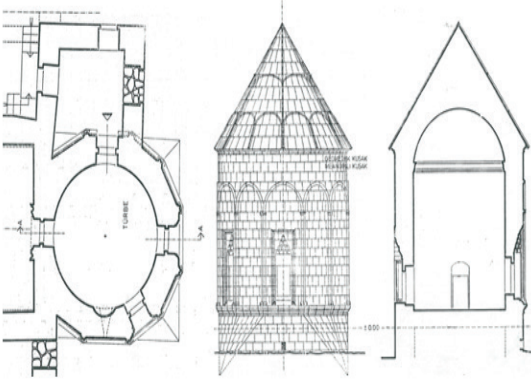
Çizim 18: Erzurum Yakutiye Medresesi Kumbeti (Tuncer, 1991)
