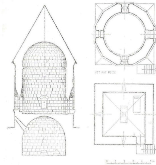
Çizim 17: Erzurum Karanlık Kümbet (Tuncer, 1991)
