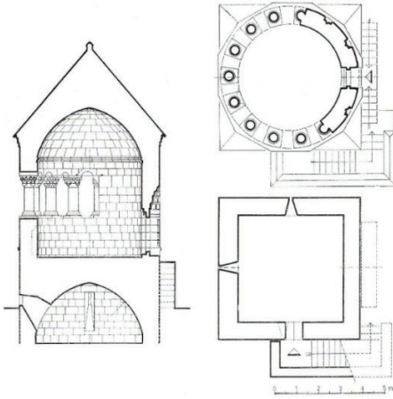
Çizim 13: Ahlat Emir Bayındır Kümbeti (Tuncer, 1991)
