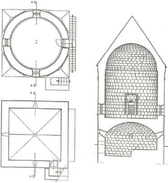
Çizim 6: itlis Güroymak Kümbeti (Tuncer, 1991)
