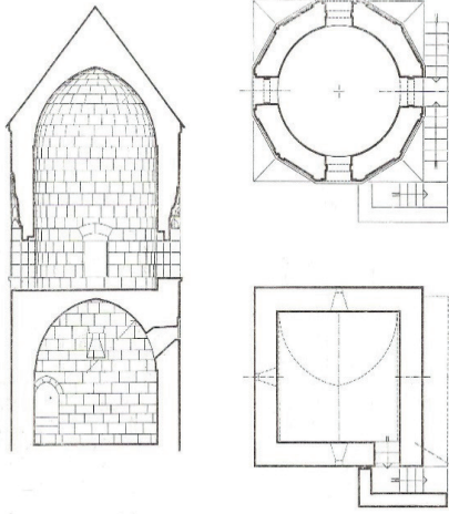
Çizim 23: Ahlat Kitabesiz Kümbet (Tuncer, 1991)
