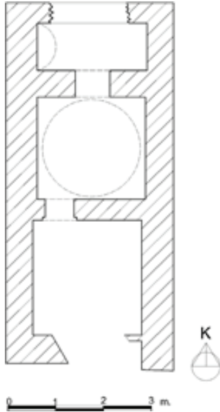
Çizim 14: Hisarköy Hamamı, plan.
