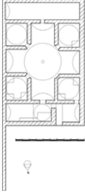
Çizim 9: Tandi’nin Hamamı, plan.
