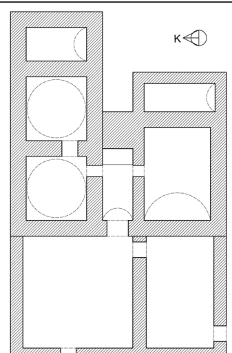
Çizim 21: Osmanlı Çeşmesi Hamamı, 3. evre.
