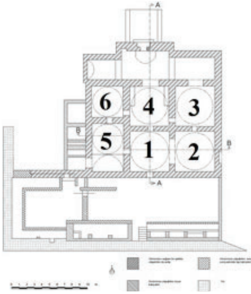
Çizim 10: Keltikli Hamam, plan.
