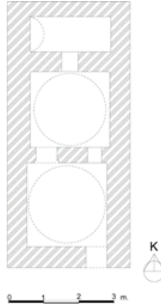
Çizim 15: Hisarköy Hamamı, restitüsyon.
