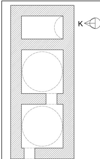
Çizim 19: Osmanlı Çeşmesi Hamamı, 1. evre.
