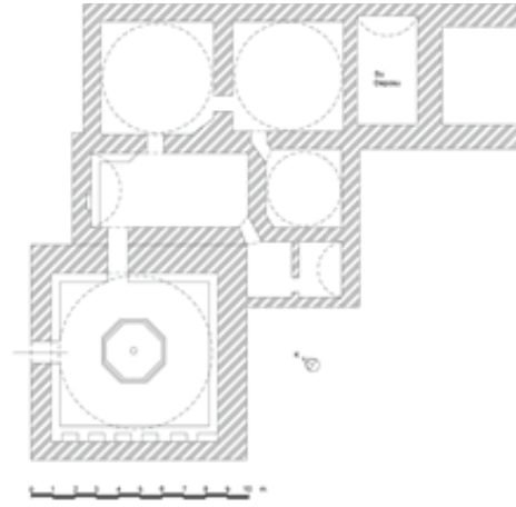
Çizim 13: Kızıl Hamam, restitüsyon.
