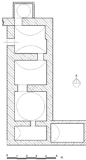
Çizim 8: Muslu Çavuş Hamamı, plan.
