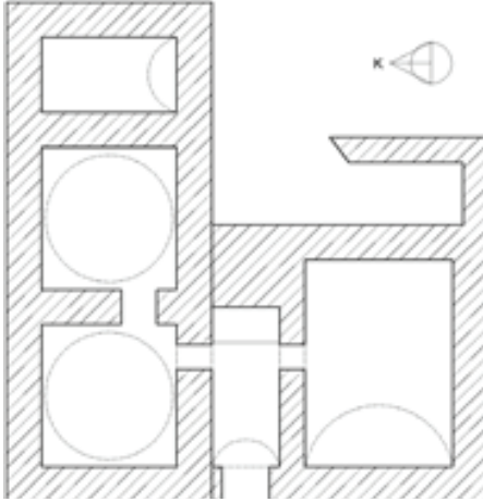
Çizim 18: Osmanlı Çeşmesi Hamamı, kroki.
