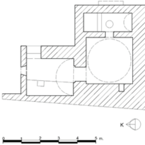
Çizim 16: Şömineli Ev Hamamı, plan.
