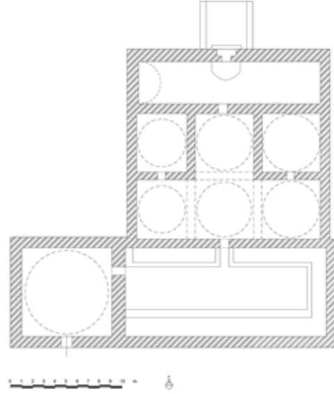
Çizim 11: Keltikli Hamam, restitüsyon.
