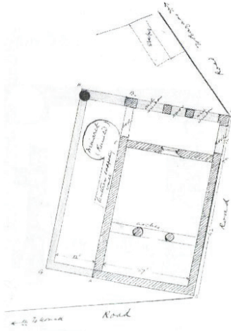
Çizim 11- Baf Yeni Cami Planı (Bağışkan'dan)
