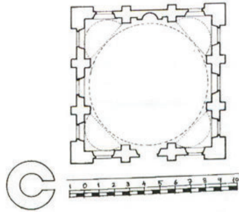
Çizim 28- Lapta Aşağı Camii Planı (Bağışkan'dan)
