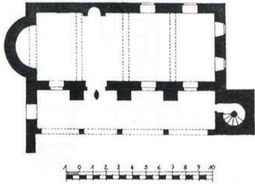
Çizim 3- Laleli Camii Planı (Bağışkan'dan)
