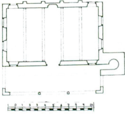
Çizim 16- Pîrî Paşa (Minareli) Camii Planı (Bağışkan'dan)
