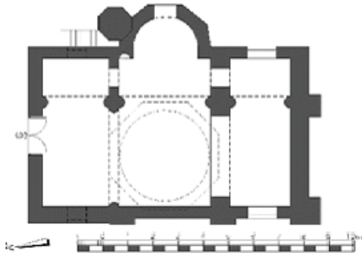
Çizim 7- Araplar Camii Planı (Çağnan'dan)
