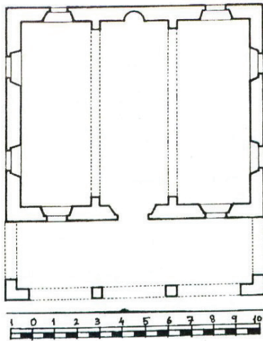
Çizim 18- Lefke Aşağı Camii Planı (Bağışkan'dan)
