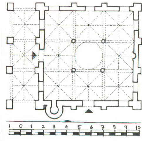
Çizim 30- Mehmetçik (Galatya) Camii Planı (Bağışkan'dan)
