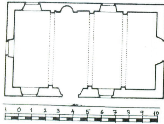
Çizim 20- Sazlıköy (Livadya) Camii Planı (Bağışkan'dan)
