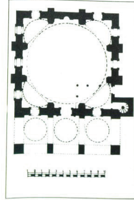
Çizim 27- Arap Ahmet Paşa Camisi Planı (Aslanapa'dan)
