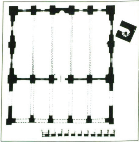
Çizim 14- Sarayönü Camii Planı (Aslanapa'dan)
