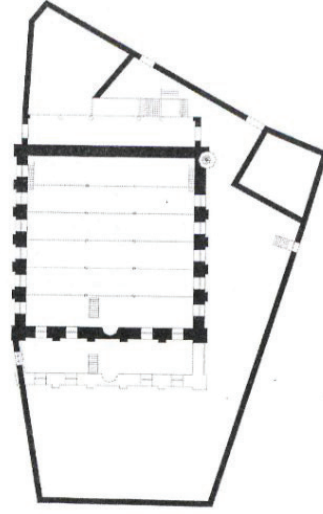
Çizim 10- Larnaka Ulu Camii Planı (Bağışkan'dan)
