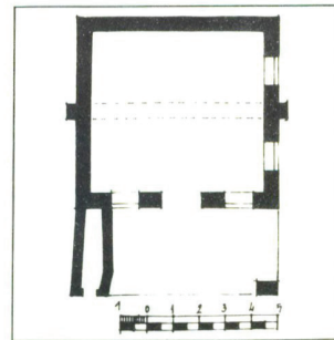
Çizim 26- Tophane Camisi Planı (Aslanapa'dan)
