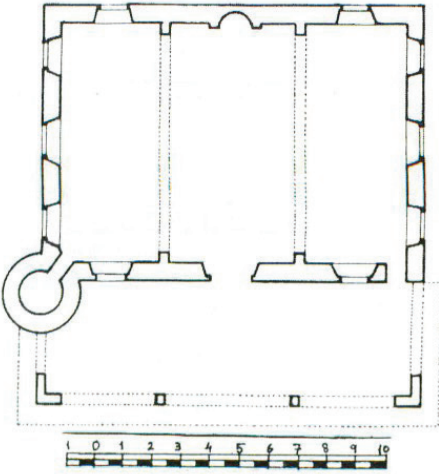
Çizim 23- Ozanköy (Kazafana) Camii Planı (Bağışkan'dan)
