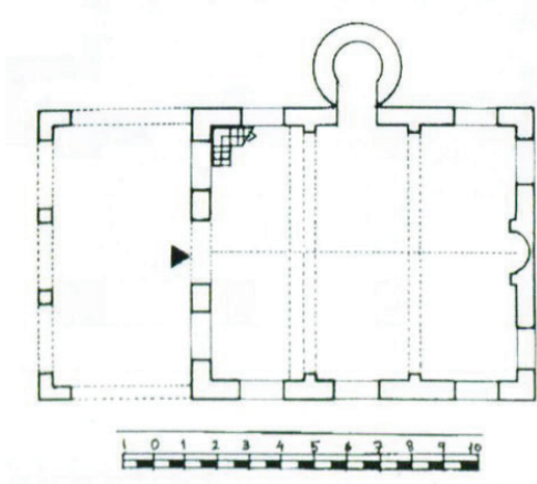
Çizim 9- İplikpazarı Camii Planı (Bağışkan'dan)
