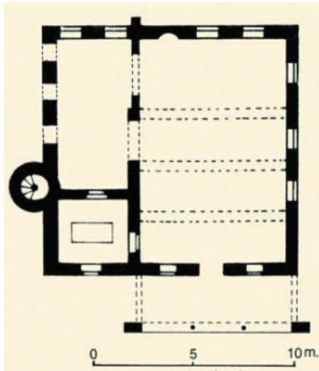
Çizim 8- Bayraktar (Şehit Alemdar) Camii Planı (Aslanapa'dan)
