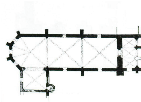
Çizim 2- Ömeriye (Ömerge) Camii Planı (Bağışkan'dan)
