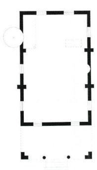
Çizim 25- Dizdarköy (Nisu) Camii Planı (Bağışkan'dan)
