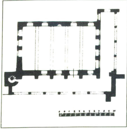
Çizim 13- Turunçlu Camii Planı (Aslanapa'dan)
