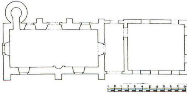
Çizim 15- Minareliköy Camii Planı (Bağışkan'dan)
